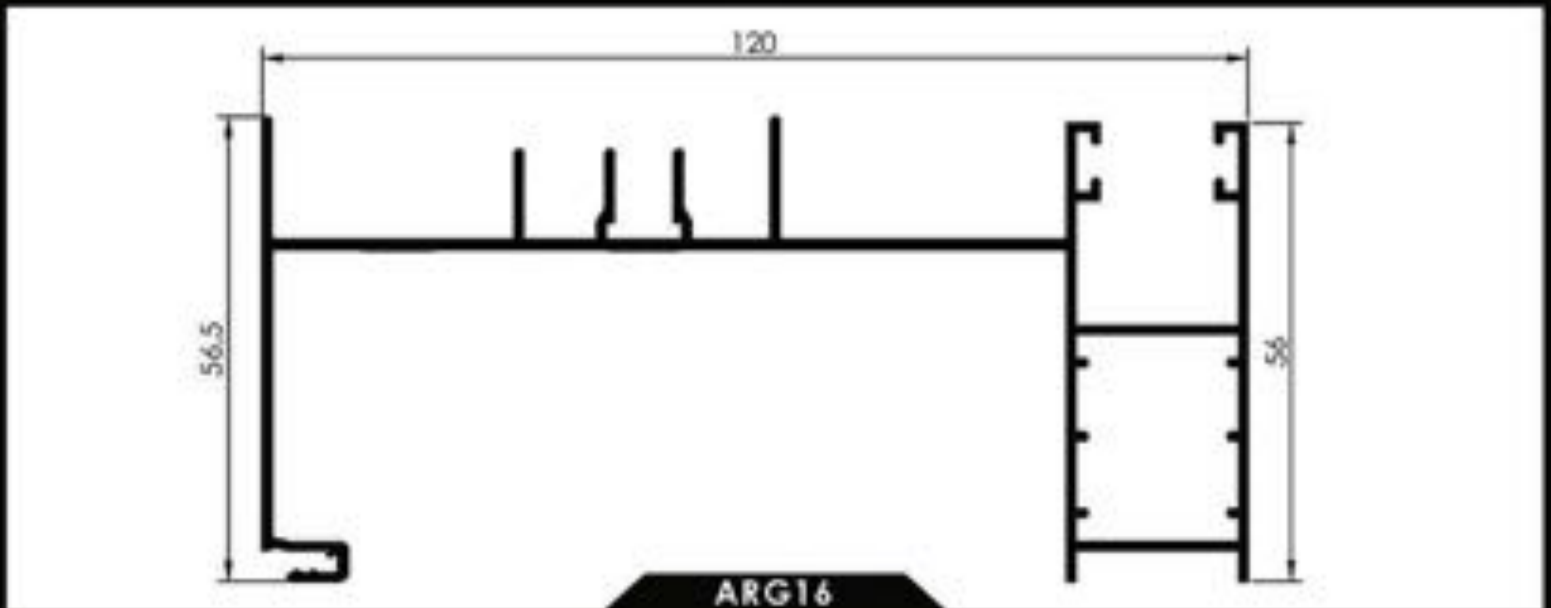
DORMANT LATERAL GAUCHE DE 120 mm
