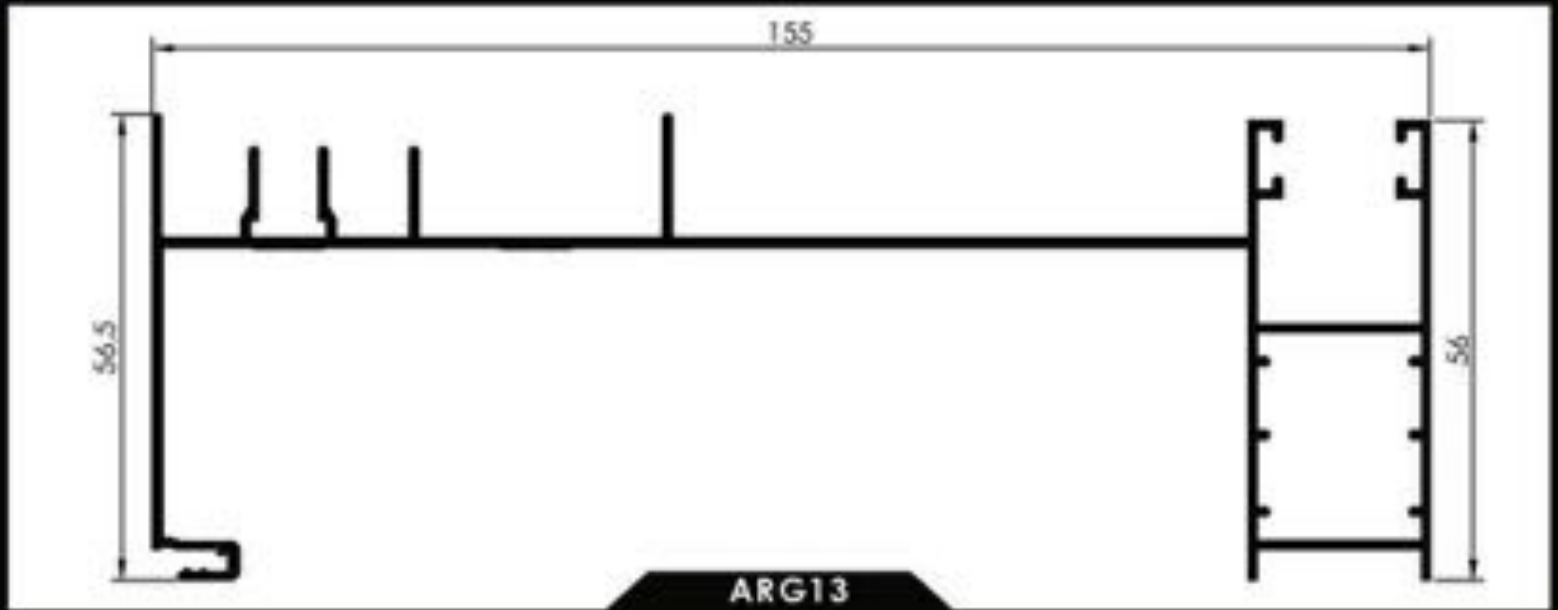
DORMANT LATERAL GAUCHE DE 155 mm
